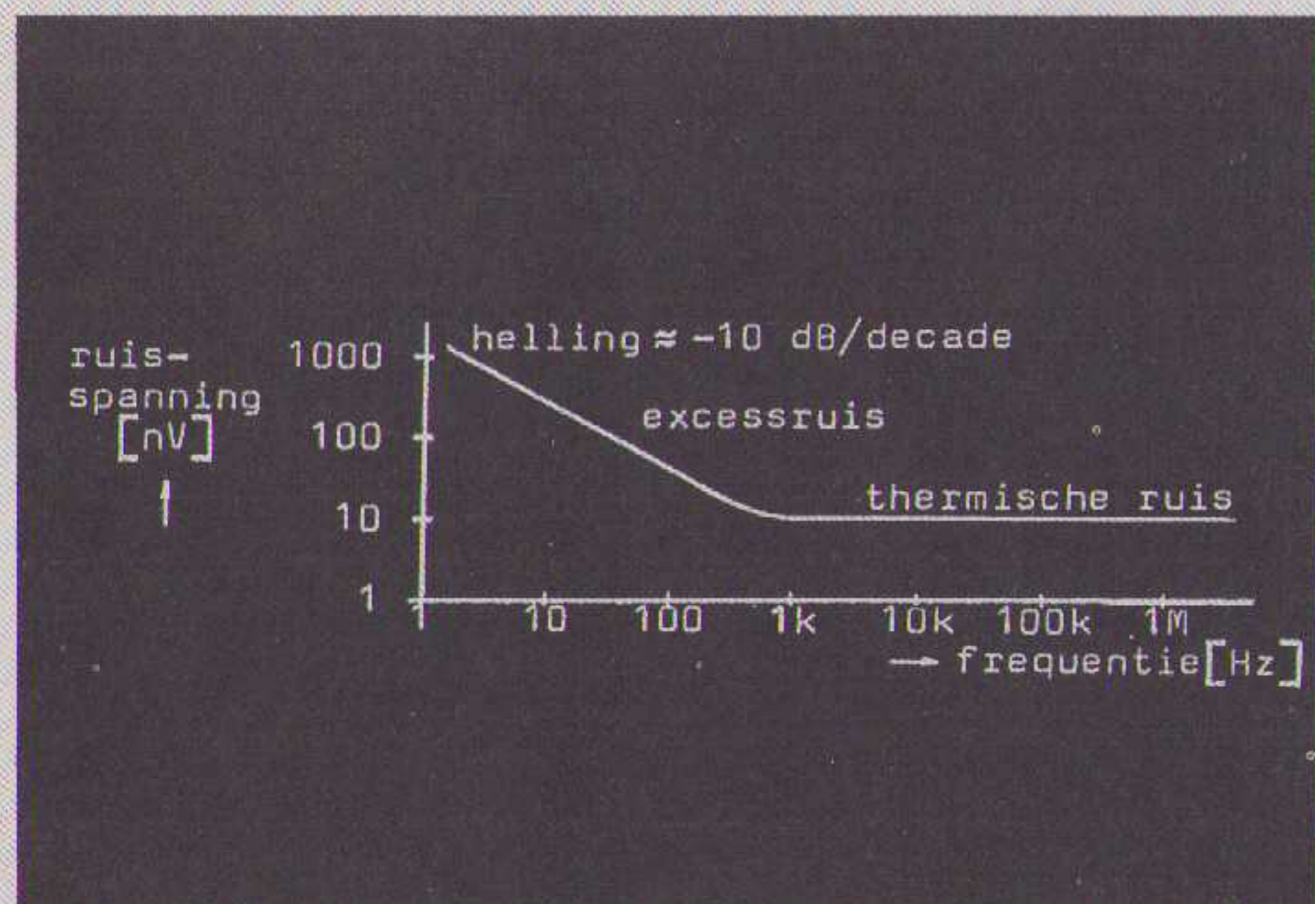
Figuur 1.3.2.2. Voorbeeld van de totale ruis spanning in een (bepaald niet ruisarme) weerstand. R = 10k , NI = 0dB en V_{DC} = 10V .
